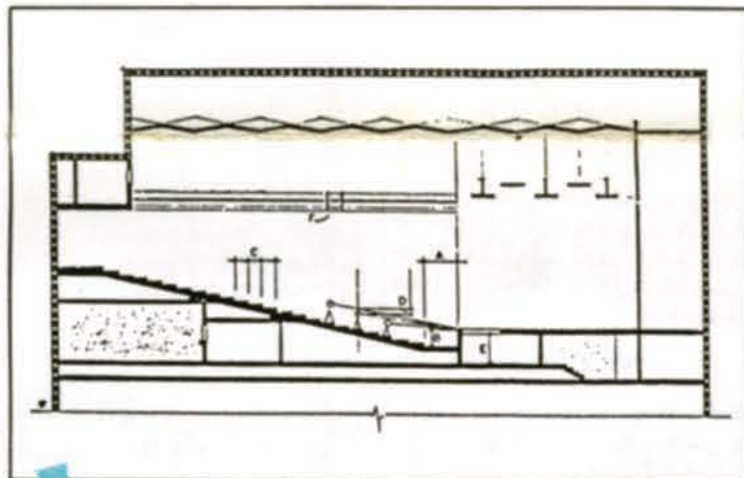
Coupe longitudinale de la salle de 800 places qui en emprise sur le métro, procurera une nouvelle vitalité à la vie musicale de Montréal ainsi qu'aux activités d'enseignement de la musique à l'UQAM.
